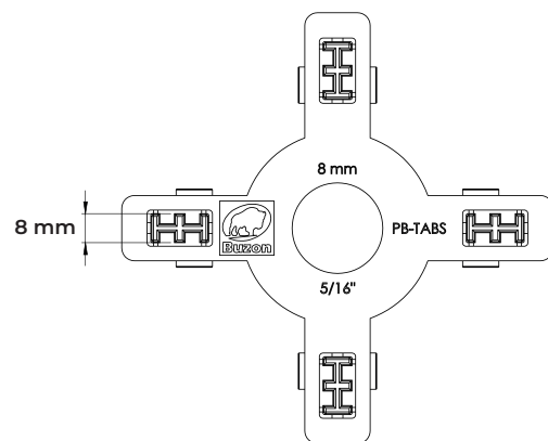
PB-TABS
