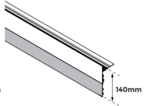
U-TFP-H80 + EXTENDER-H60
