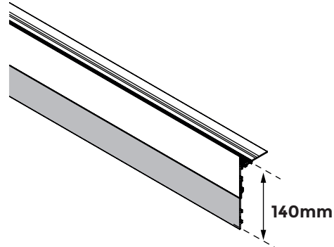
U-TFP-H80 + EXTENDER-H60
