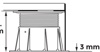
PB-3 90-145 mm
