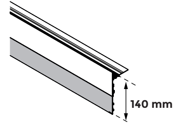
U-TFP-H80 + EXTENDER-H60
