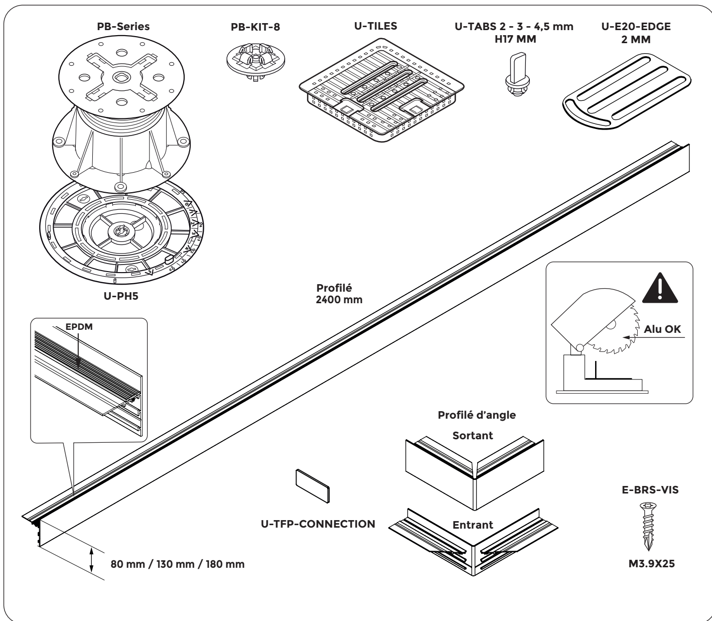
H.80 mm / PB-01
